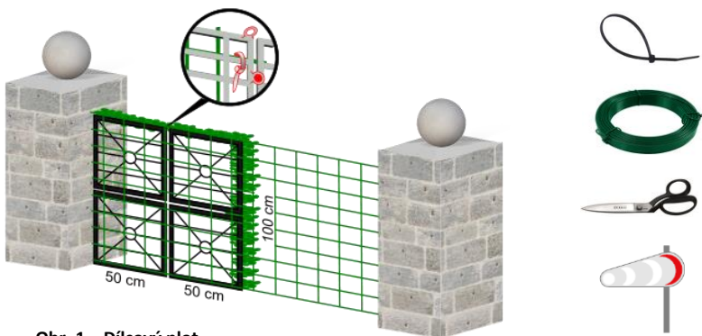
Obr. 1 – Dílcový plot
